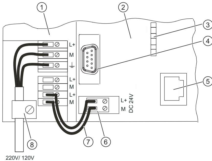
Figura 2-2 Cablear fuente de alimentación y CPU/PB-Link (tapas frontales abiertas).
